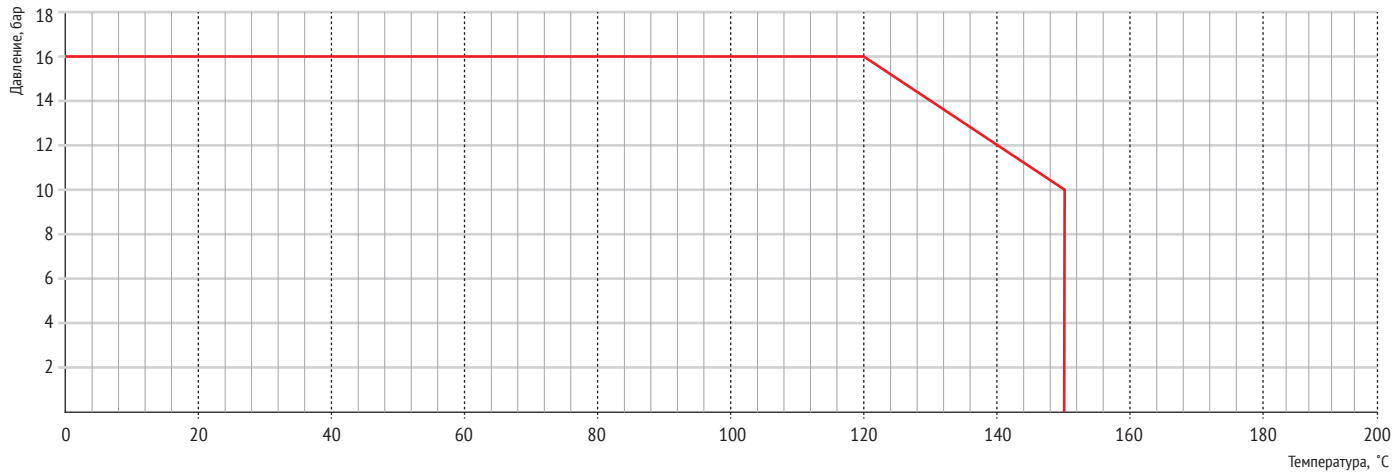
График зависимости давления от температуры.
