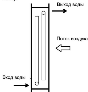
Рис.6 Водяной калорифер
