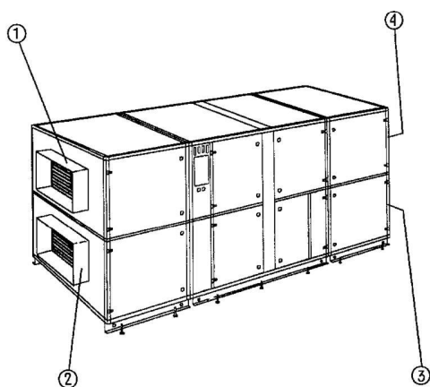
Рис.9 Измерение давления воздуха
