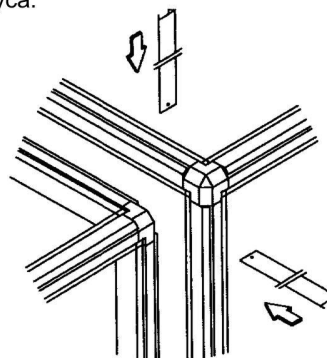
Рис.4 Сборка модулей
