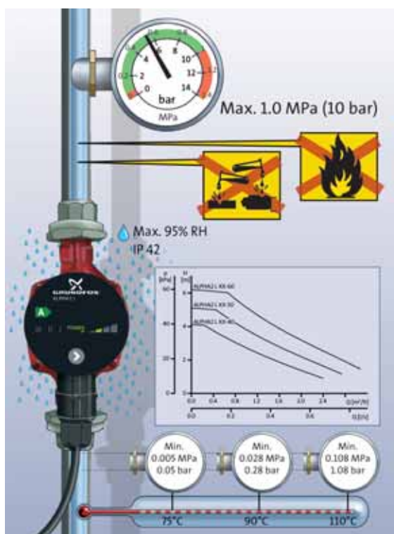
Рис. 2 Перекачиваемые жидкости и условия эксплуатации
