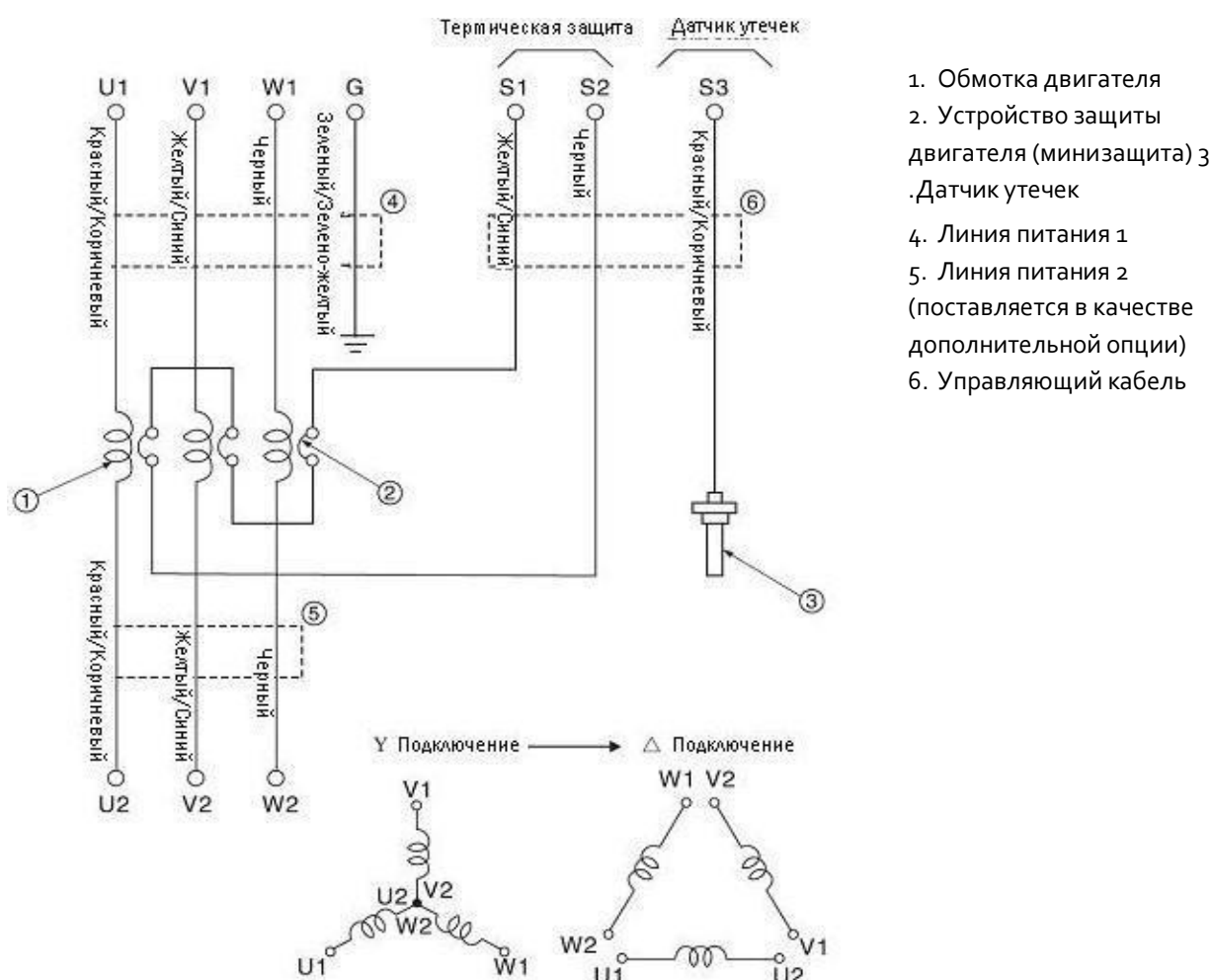
Рис. 13 Электрическая монтажная схема включения звезда и треугольник
