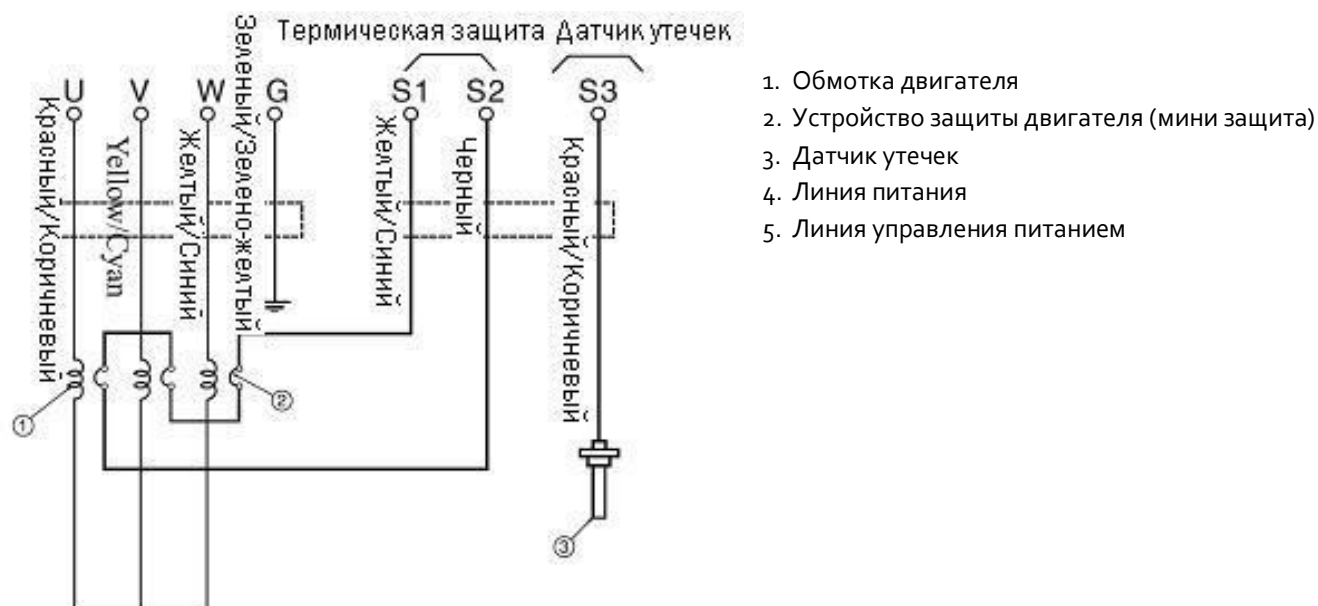
Рис. 12 Электрическая монтажная схема прямого включения (2)
