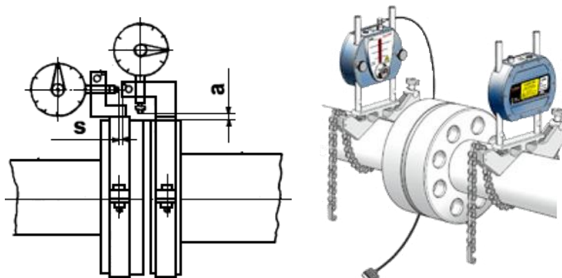
Индикаторное приспособление
