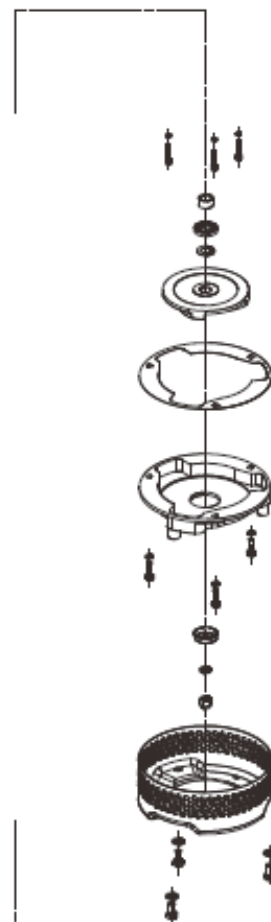
Рис. 27. МОДЕЛЬ 2: 1,5 ~ 5,5 кВт в разобранном виде
