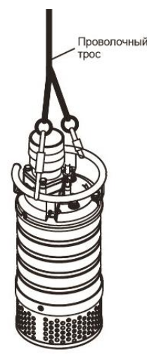
Рис.3 Подвешивание насоса
