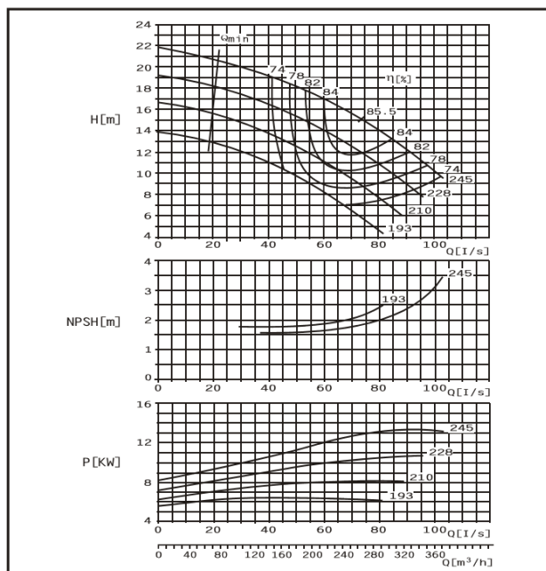
DMC125-230 E
