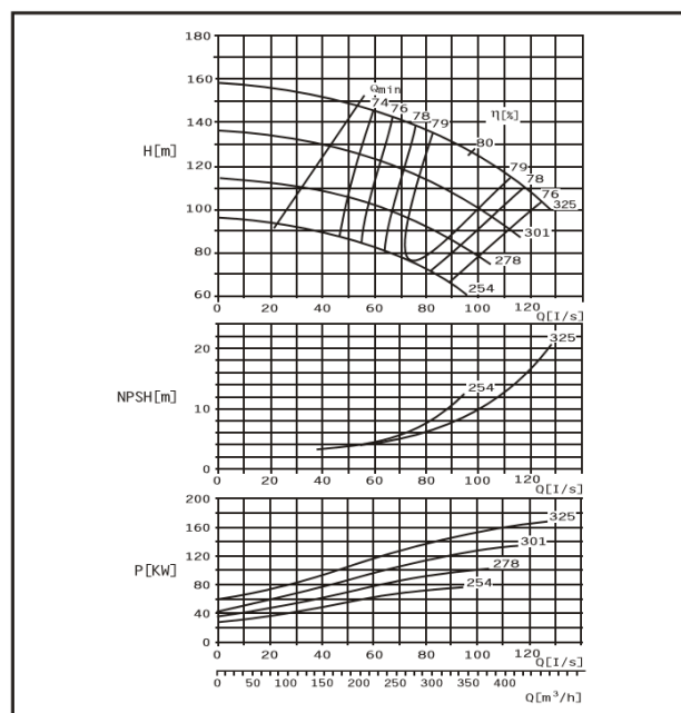
DMC100-310 EG
