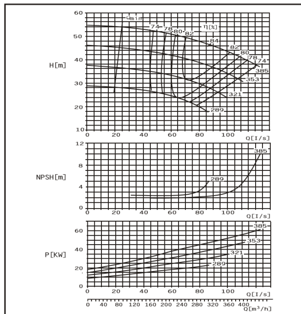
DMC125-365 E
