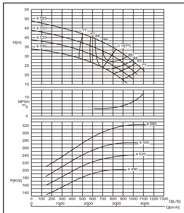
DMC500-640 F
