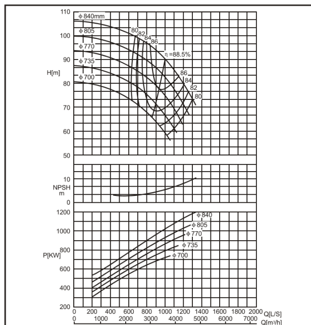
DMC500-890 F
