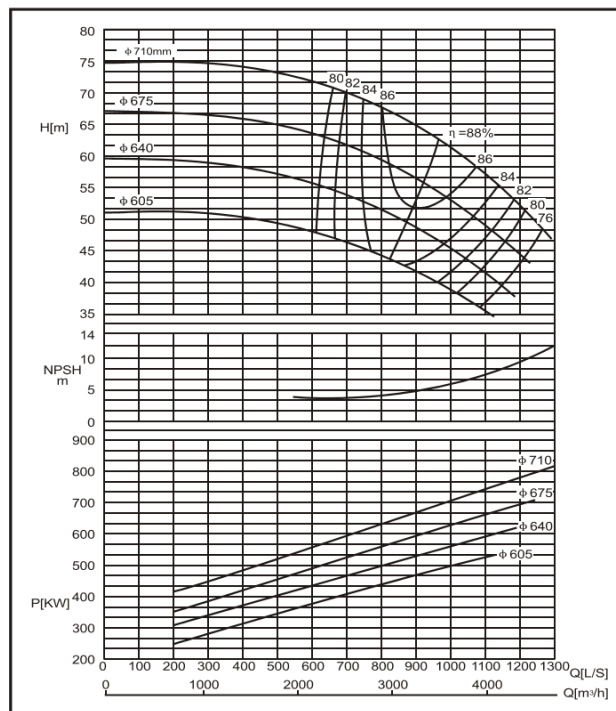
DMC500-790 F
