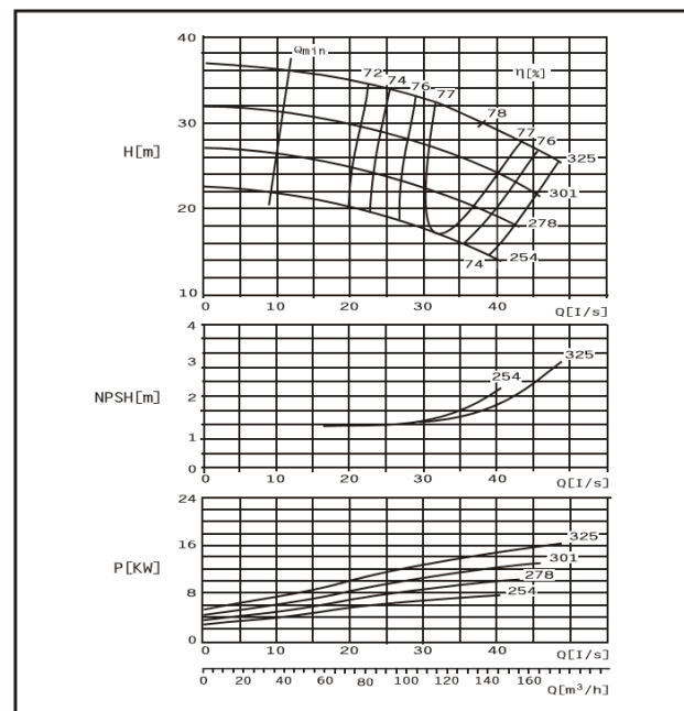
DMC100-310 F
