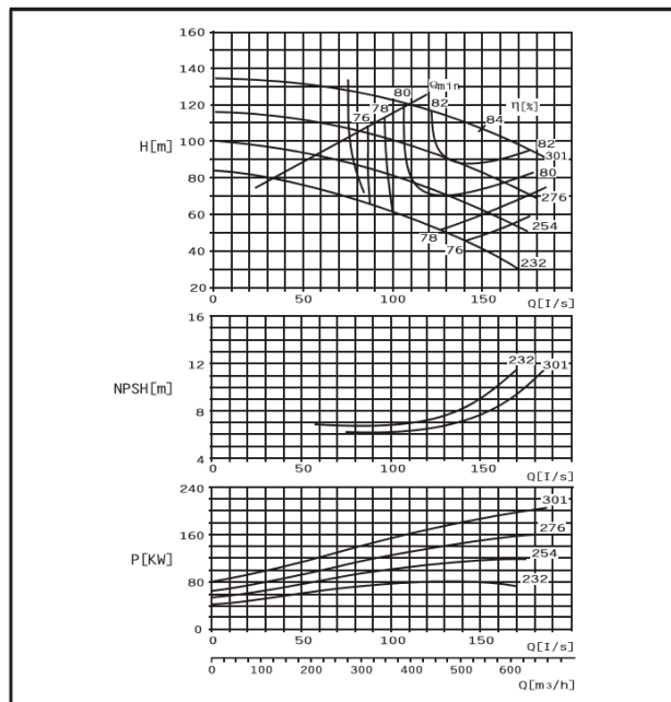
DMC125-290 EG
