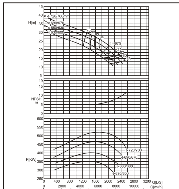
DMC800-740 F
