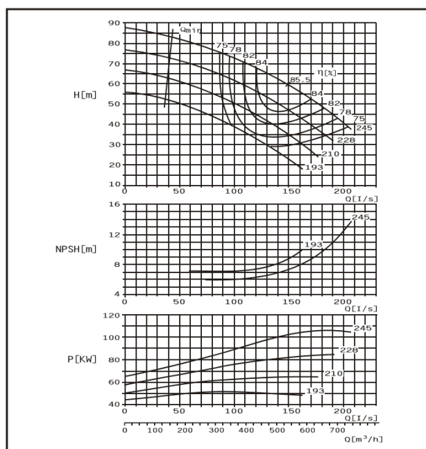
DMC125-230 EG
