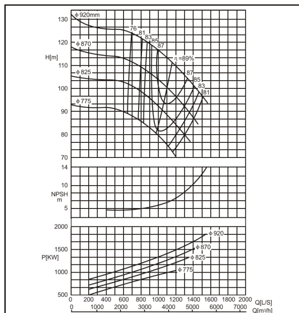
DMC500-890 E
