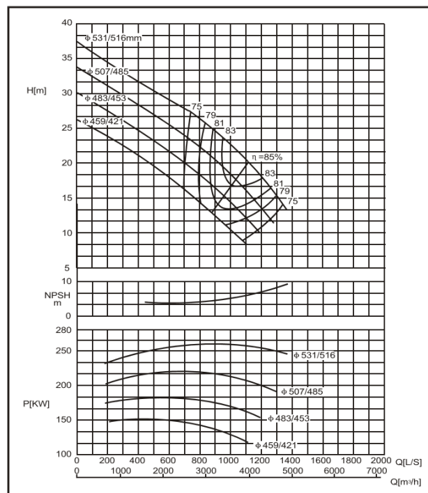
DMC600-540 F
