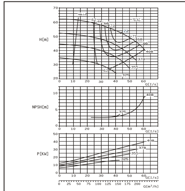
DMC100-375 F
