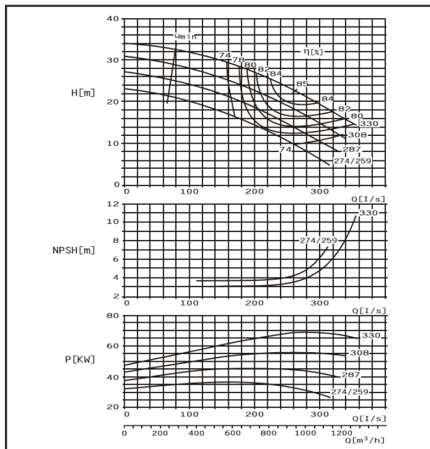
DMC300-300 F
