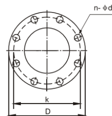
Фланец
