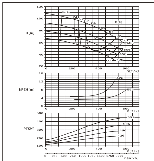
DMC300-560 F
