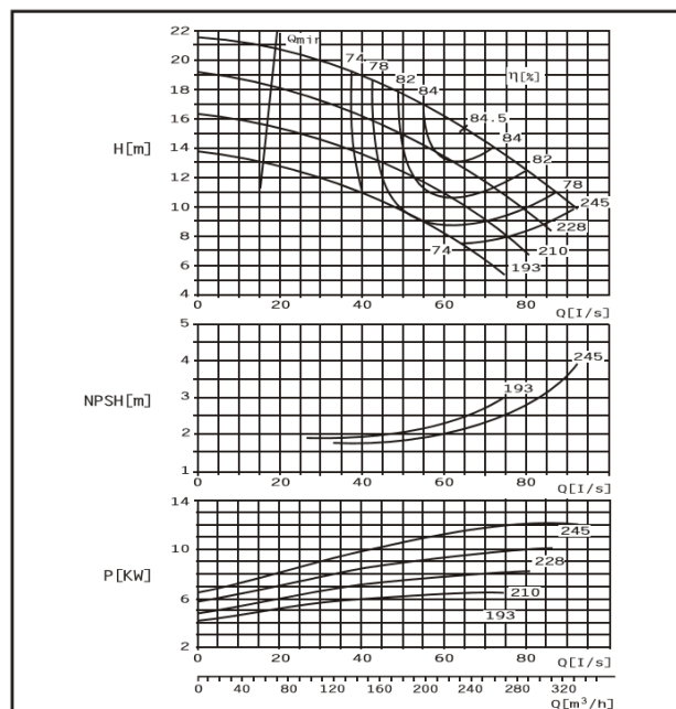
DMC125-230 F
