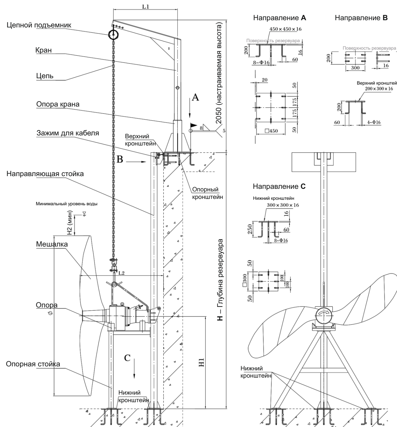
Рисунок 7 — Схема системы установки типа IV
