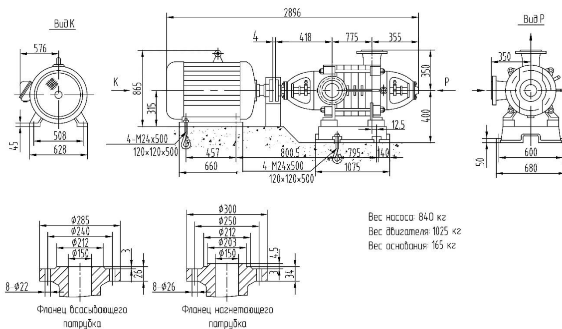
Габаритные размеры D155-30x6
