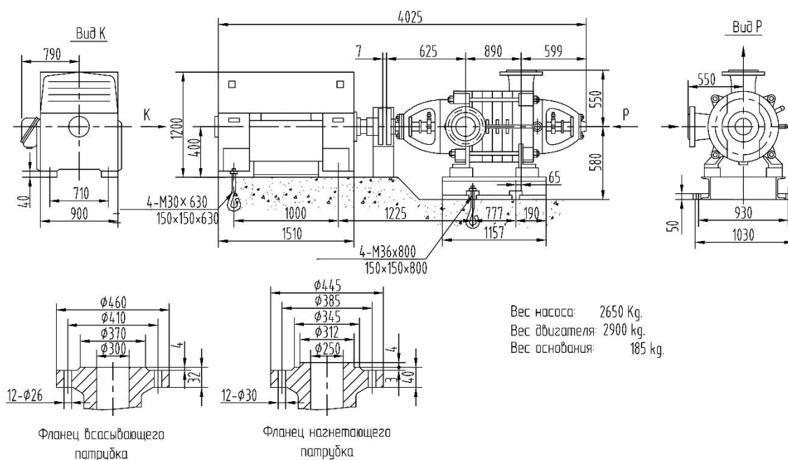
Габаритные размеры D600-60x4
