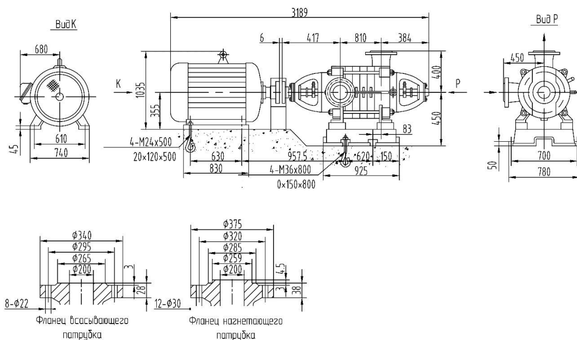
Габаритные размеры D360-40x5
