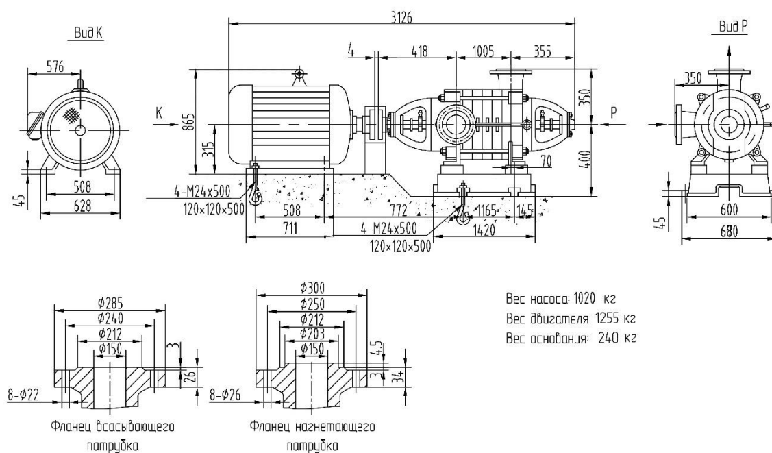
Габаритные размеры D155-30x8
