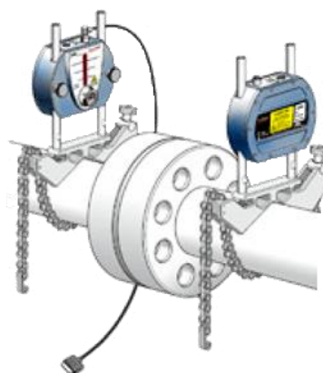
Прибор лазерной центровки
