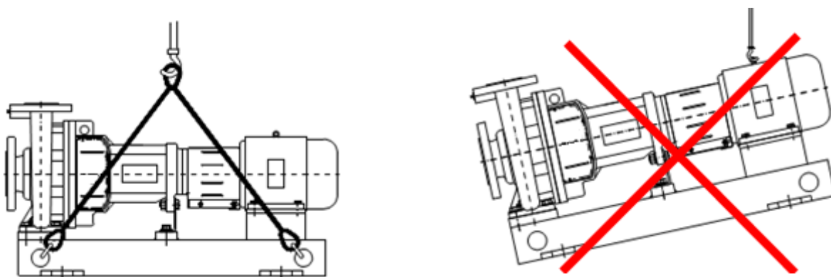
Рисунок 1 Схема строповки агрегата электронасосного серии HSC
