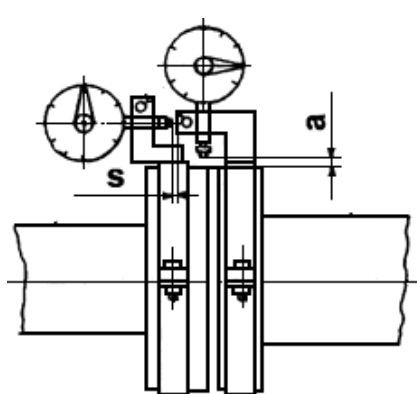
Индикаторное приспособление
