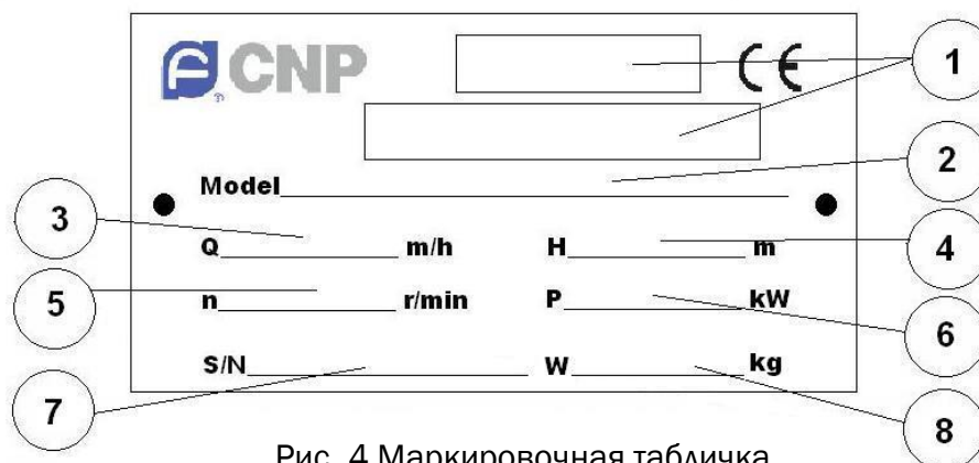
Рис. 4 Маркировочная табличка
