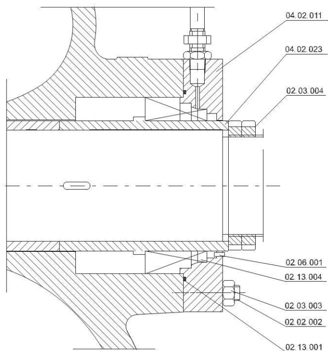
Рис. 17 Механическое уплотнение тип А к горизонтальным насосам типа А и В
