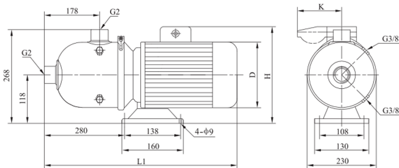
Габаритно-присоединительные размеры
