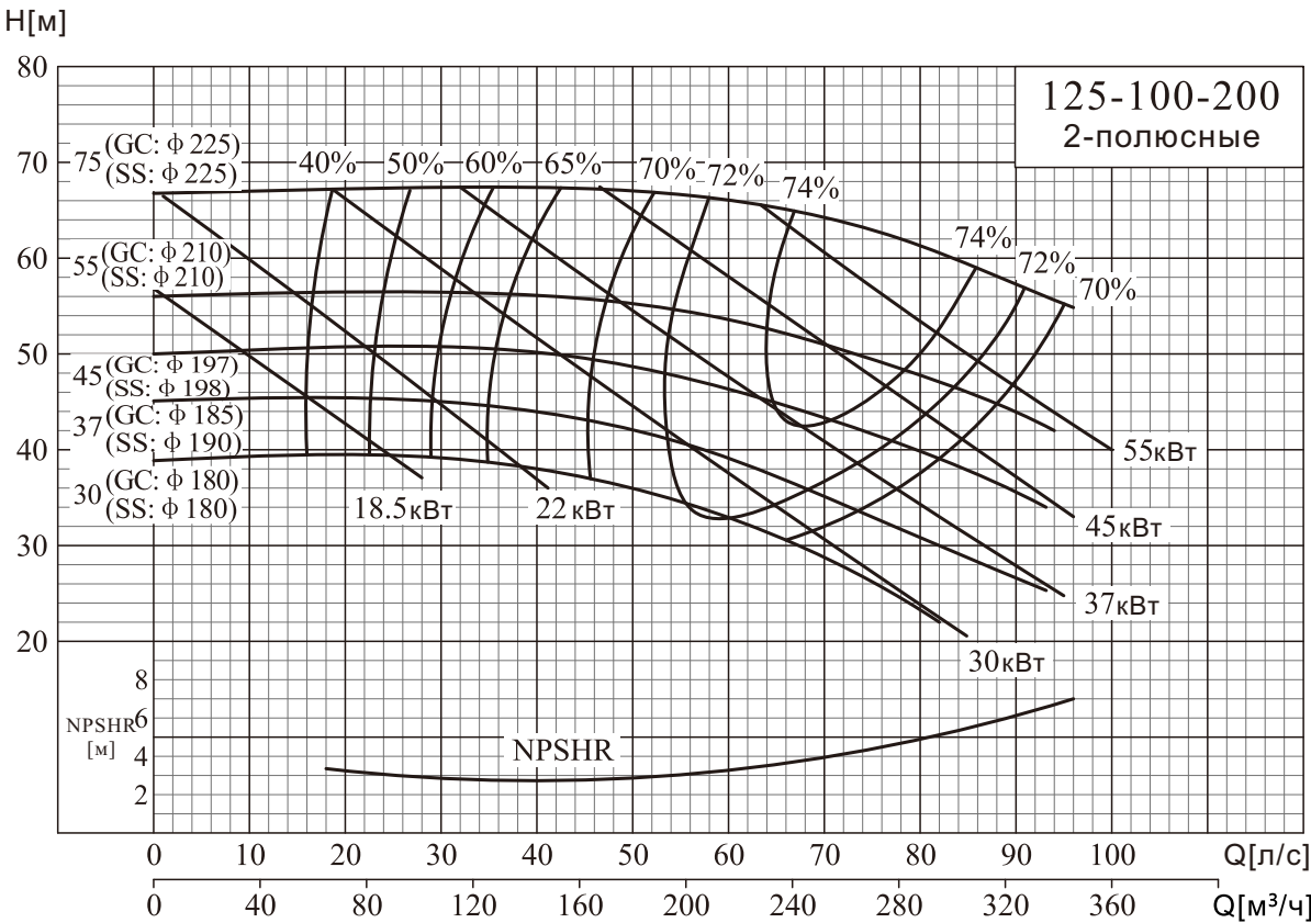
NISO,NIS,NISF125-100-200/125-100-250
