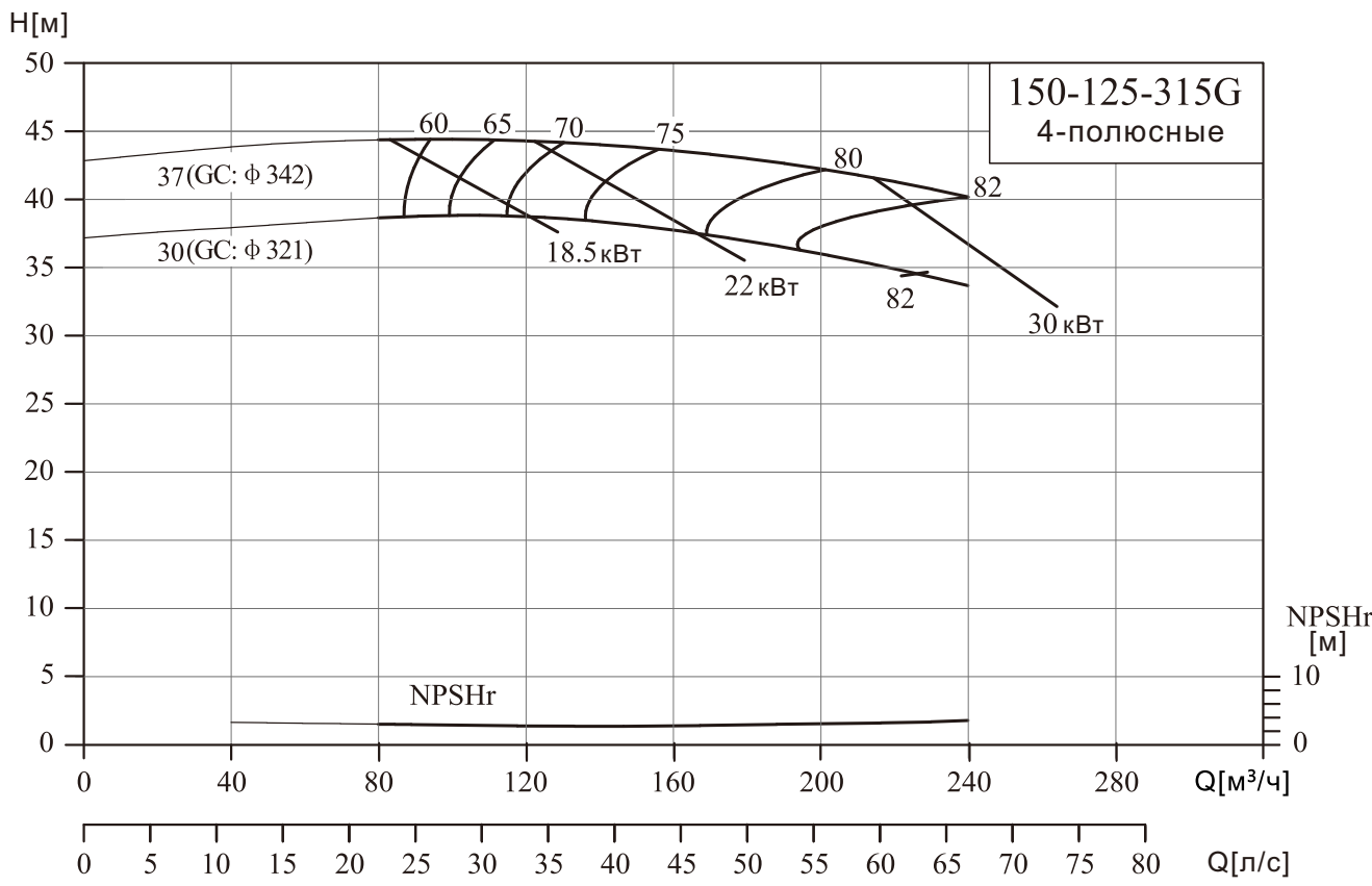
NIS150-125-315G/150-125-400(Q)
