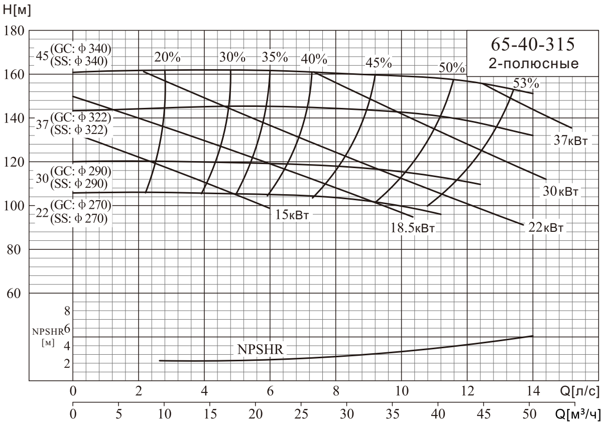
NISO,NIS,NISF 65-40-315/65-50-160
