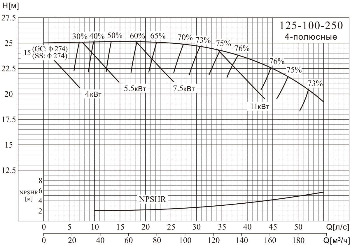
NISO,NIS,NISF 125-100-250/125-100-315
