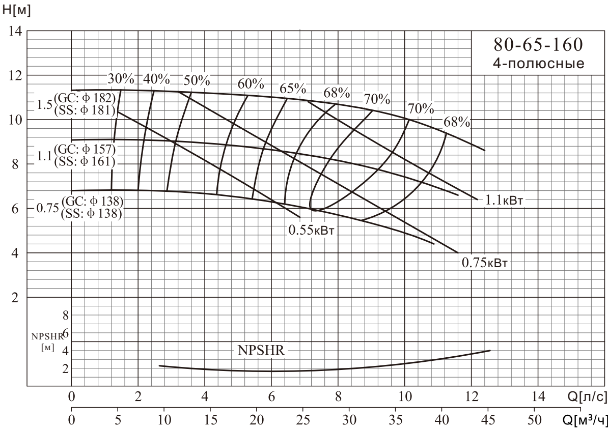
NISO,NIS,NISF 80-65-160/100-65-200
