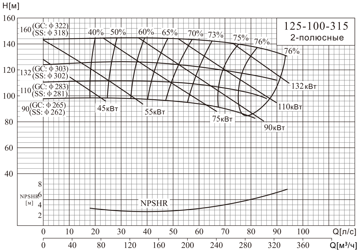
NISO,NIS,NISF 125-100-315/50-32-160
