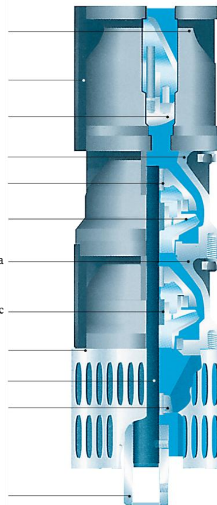
Рисунок 14. Структура насосной части погружного агрегата насосного SJ
