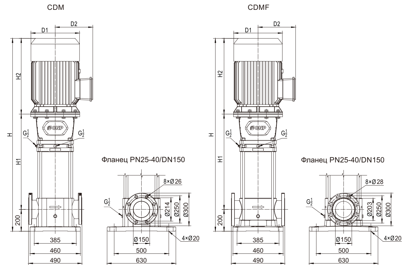
Габаритно-присоединительные размеры однофазного электродвигателя и взрывозащищенного двигателя имеют небольшие отличия. Пожалуйста, обратитесь в представительство в вашем регионе для уточнения.
