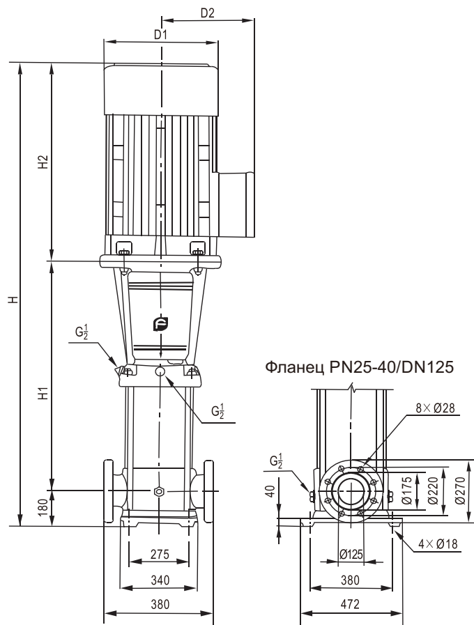
Габаритно-присоединительные размеры однофазного электродвигателя и взрывозащищенного двигателя имеют небольшие отличия. Пожалуйста, обратитесь в представительство в вашем регионе для уточнения.
