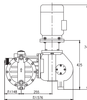
RX700-1200 металлическая проточная часть спереди
