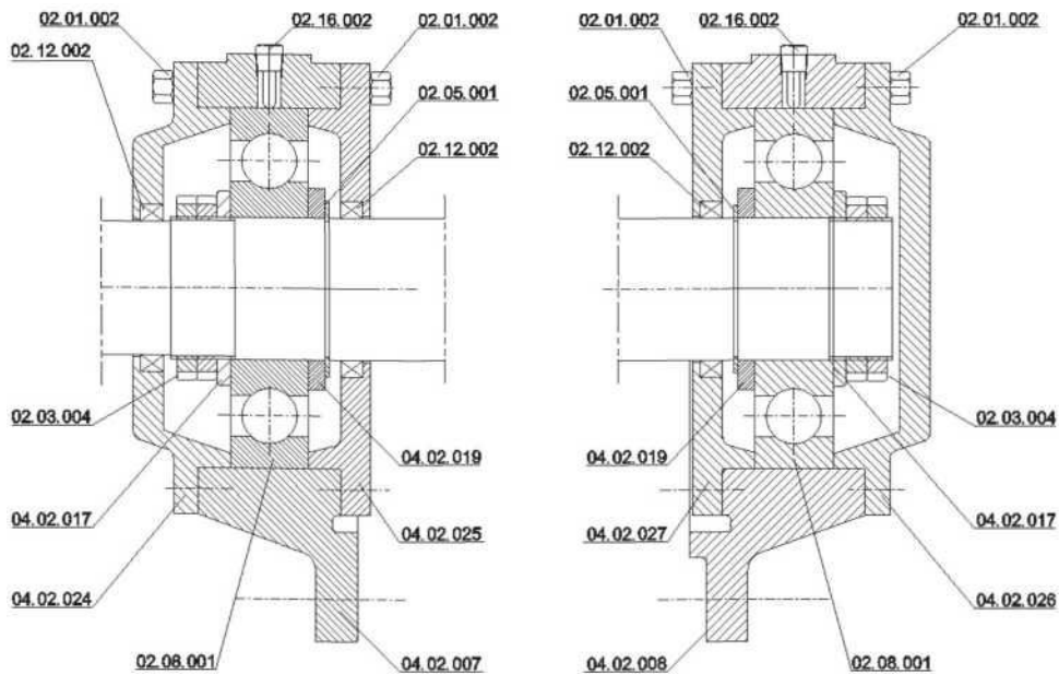
Тип А—Применяется в горизонтальных установках тип А
