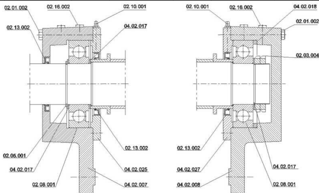
Тип С—Применяется в горизонтальных установках тип С
