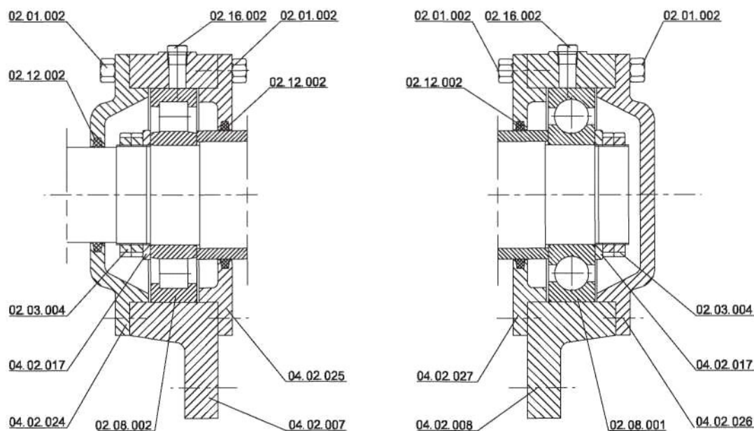
Тип В—Применяется в горизонтальных установках тип В
