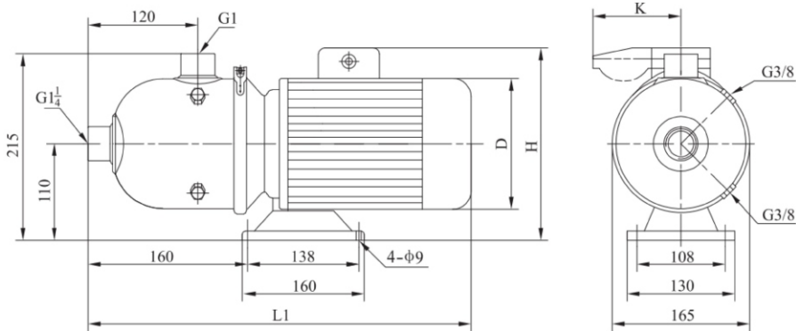
Габаритно-присоединительные размеры и масса
