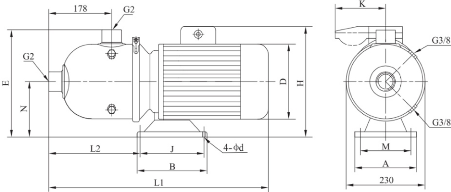
Габаритно-присоединительные размеры и масса
